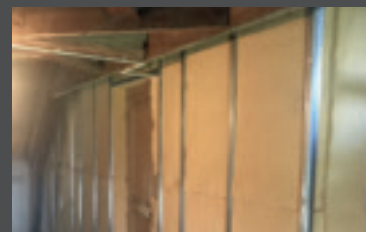
ISOLATION DES MURS ET RAMPANTS EN PANNEAUX DE FIBRES DE BOIS À GRIÈGES
